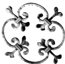
Ø 250 mm ⌀ 8 x 8 mm con fascette/with collars Art. 20/5 senza fascette/without collars Art. 20/6 Art. 186/2 Zincato a caldo Hot galvanized
